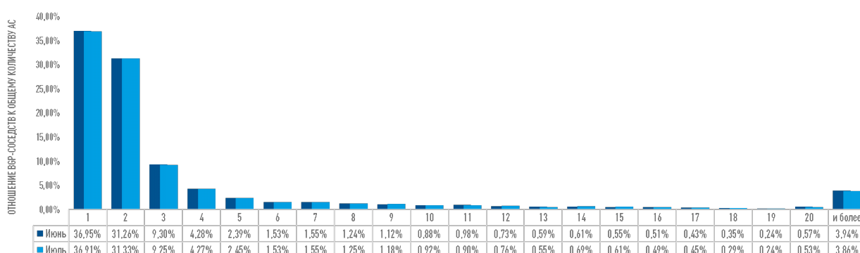
Связность автономных систем в июне и июле 2025 года
